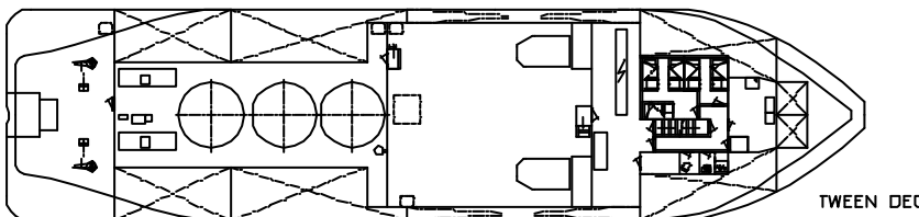
TWEEN DECK
